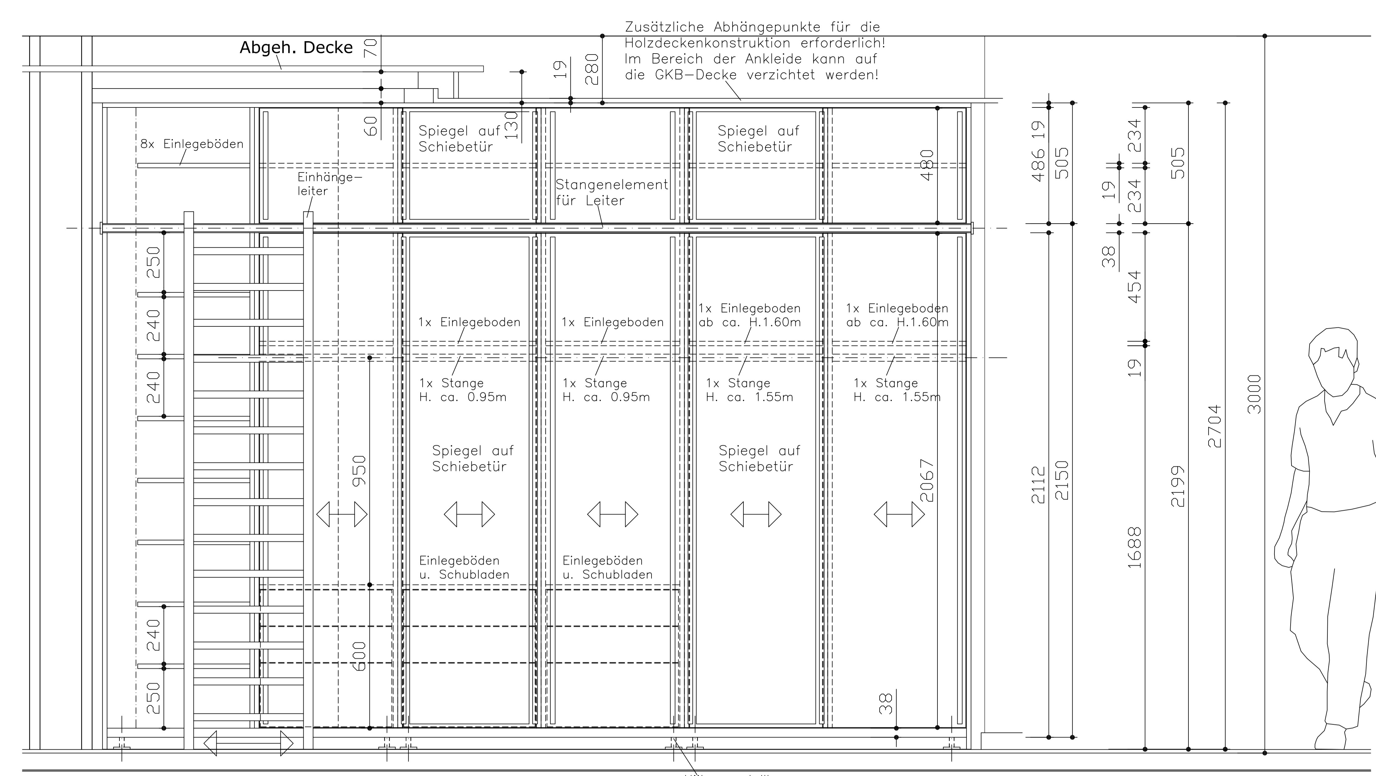
ANSICHT Schrank 3
