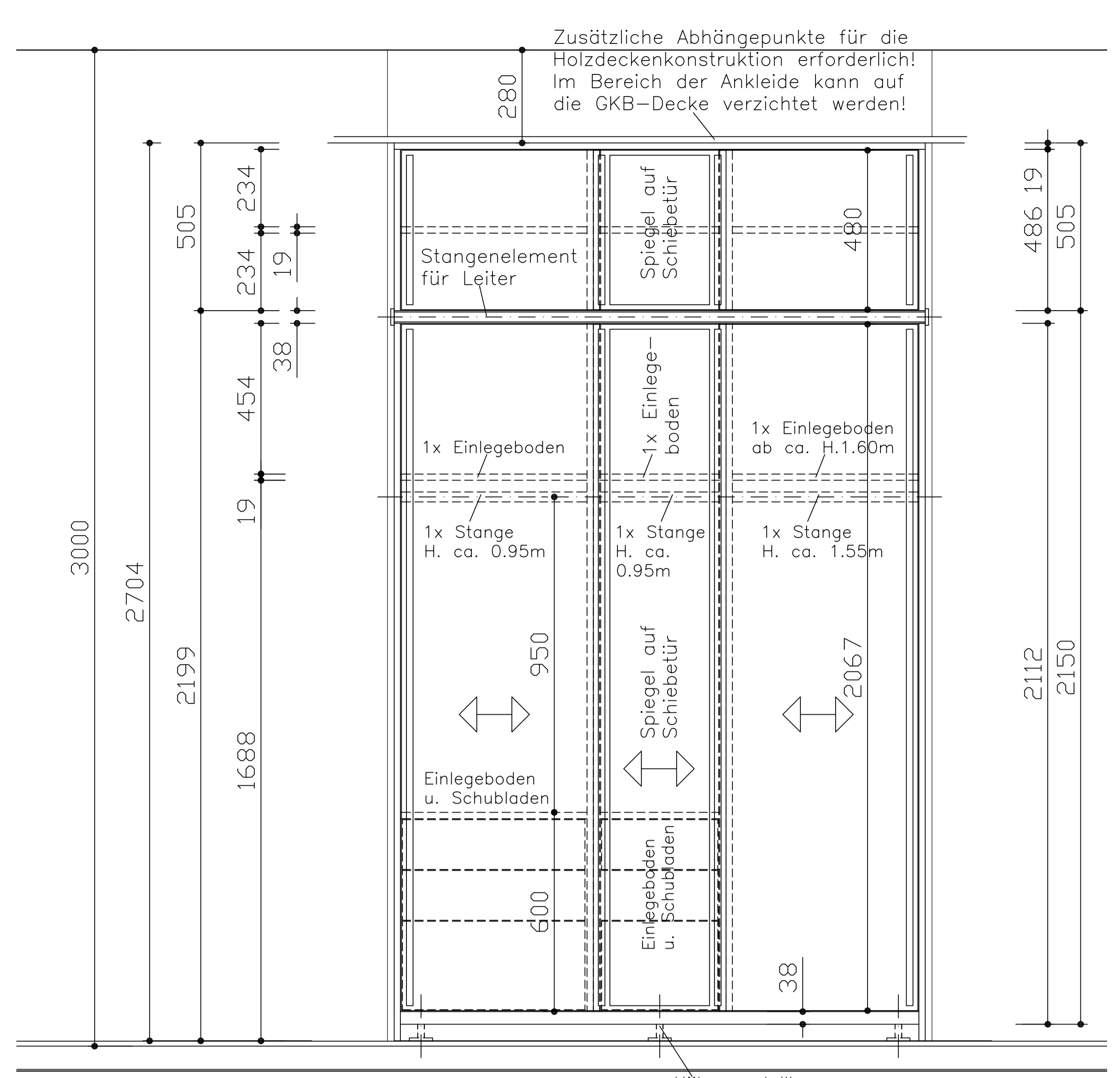
ANSICHT Schrank 2
